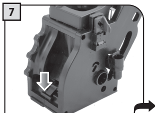
7 Dźwignia położona w części tylnej, musi znajdować się w kontakcie z podstawą zespołu.
