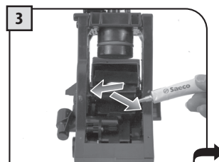
3 Smarować prowadnice zespołu jedynie smarem dostarczonym w wyposażeniu.
