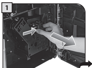
1 Nacisnąć przycisk PUSH, aby wyciągnąć Blok Kawy.
